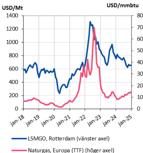
Figur 20. Priset på lågsavvlig marindiesel (LSMGO i Rotterdam) samt Naturgas (TTF) januari 2018 – mars 2025.
