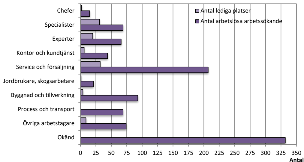
Figur 3: Antal arbetslösa arbetssökande efter yrke, den 15 maj 2020
