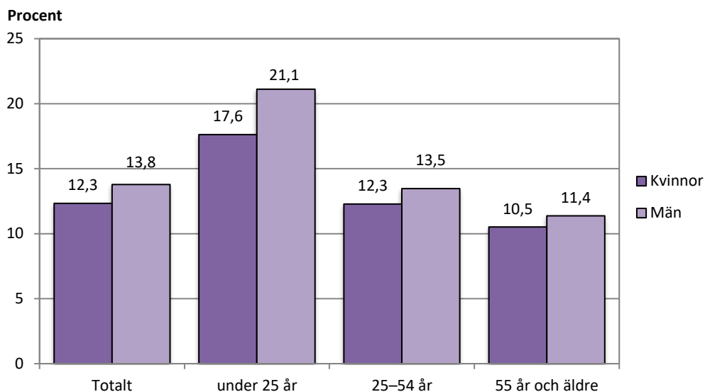
Figur 4: Det relativa arbetslöshetsstalet efter ålder och kön (%) den 15 maj år 2020
