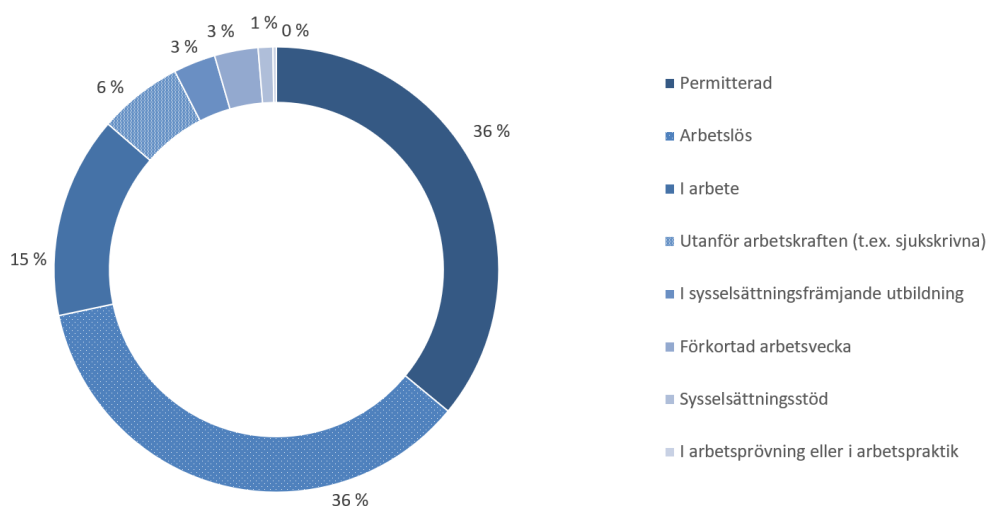
Figur 1: Arbetssökande personer den 15 maj efter arbetsmarknadsstatus
