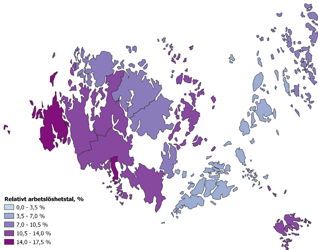
Figur 5: Det relativa arbetslöshetstalet den 15 maj efter kommun (procent)
