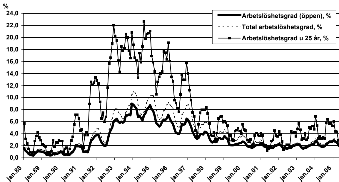
Figur 1: Arbetslöshetsgrader januari 1988 - juli 2005
