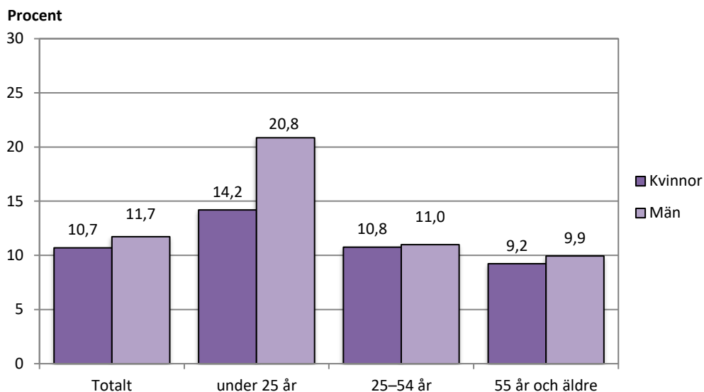
Figur 4: Det relativa arbetslöshetsstalet efter ålder och kön (%) i juli år 2020
